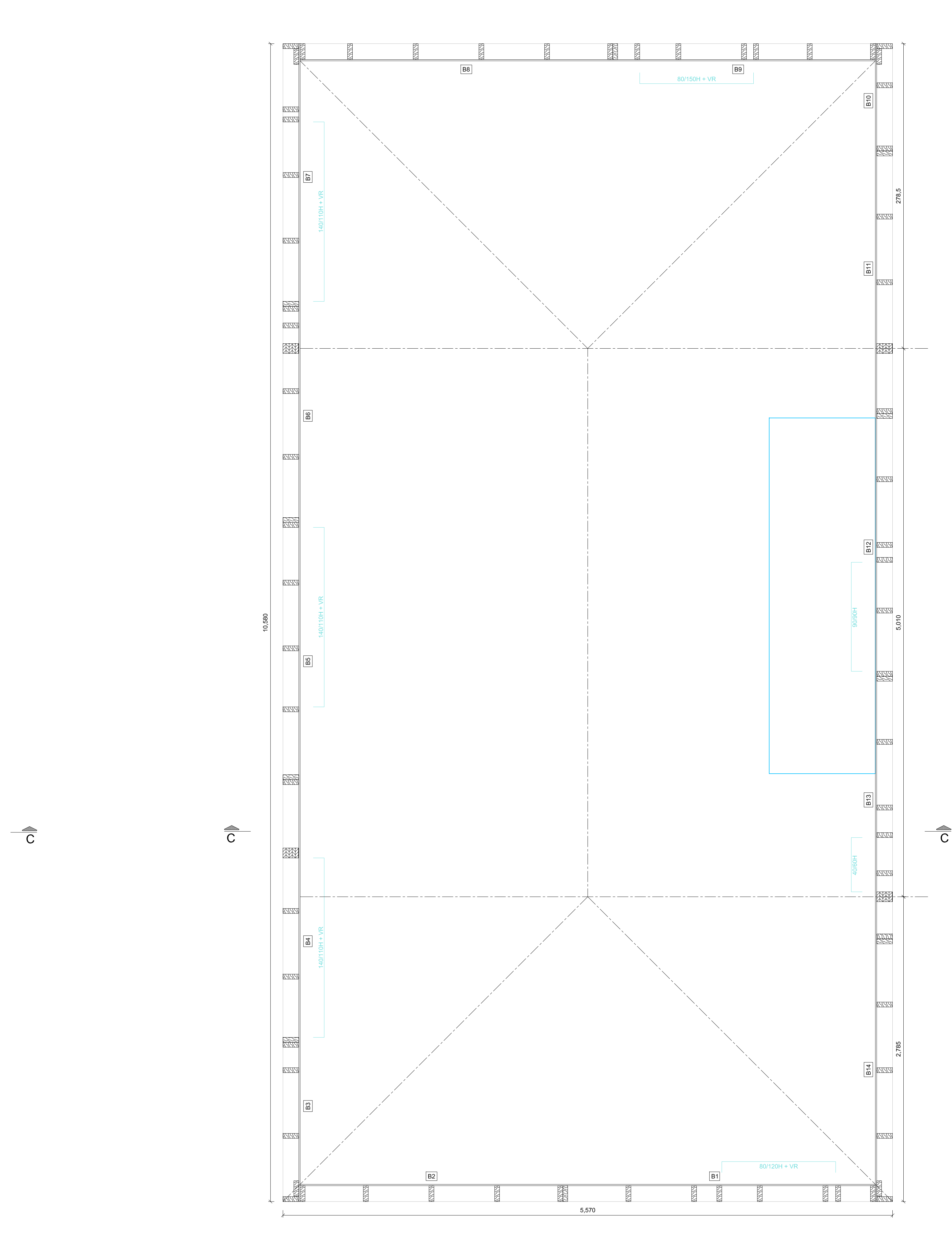
Murs bois étage - Implantation & nomenclature ech.1/20
