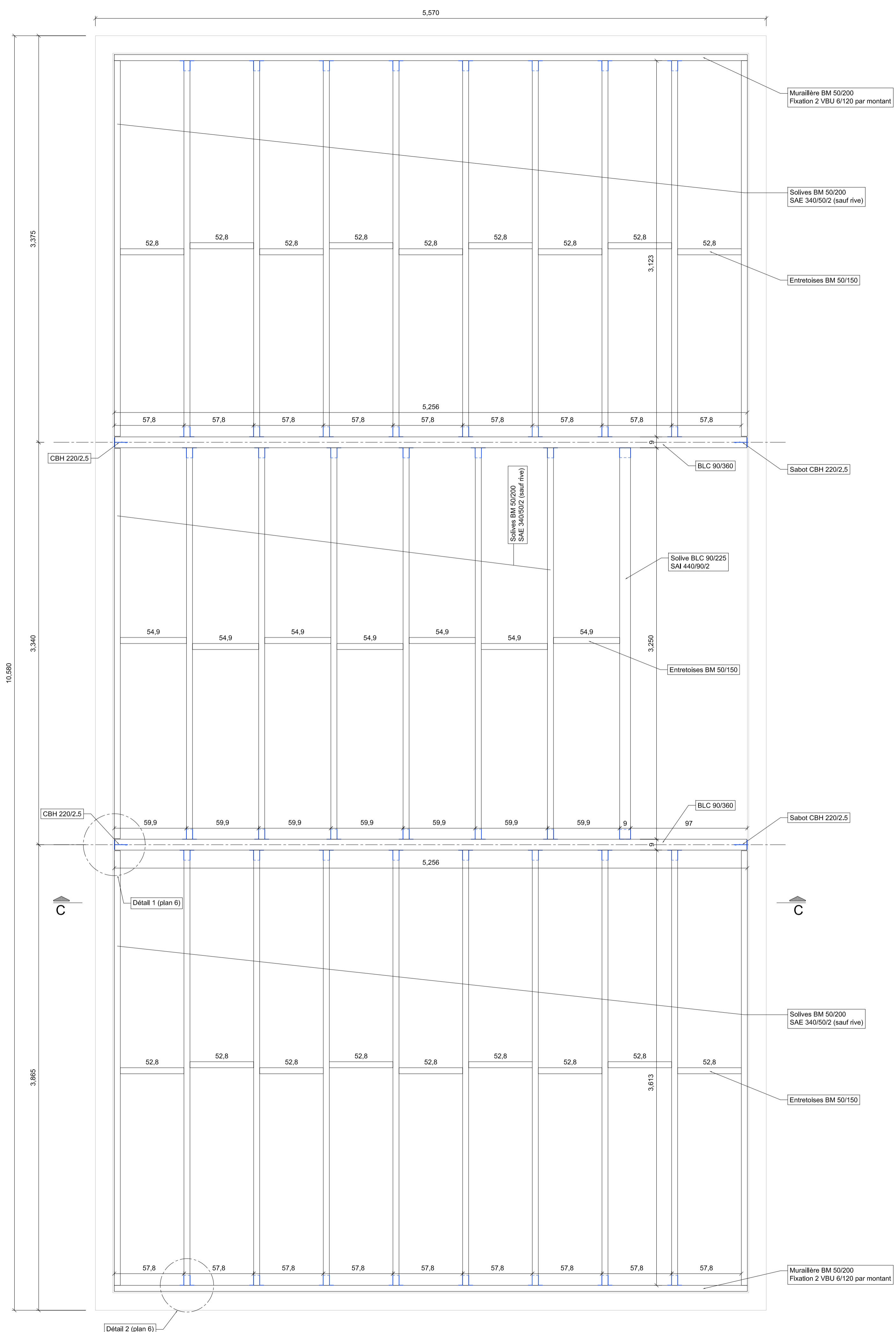
Solivage R+1 - Vue en plan ech.1/20
